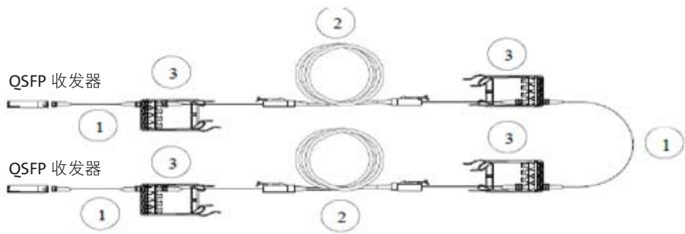
图 12: 交叉互联结构化布线的多光纤并行连接
