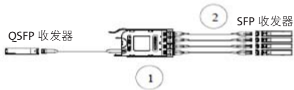
图 16: 使用带尾纤模块的 8 芯到 2 芯互联结构化布线
