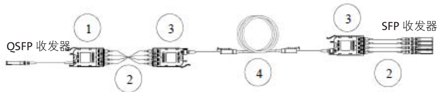
图 18: 使用带尾纤模块的 8 芯到 2 芯交叉互联结构化布线
