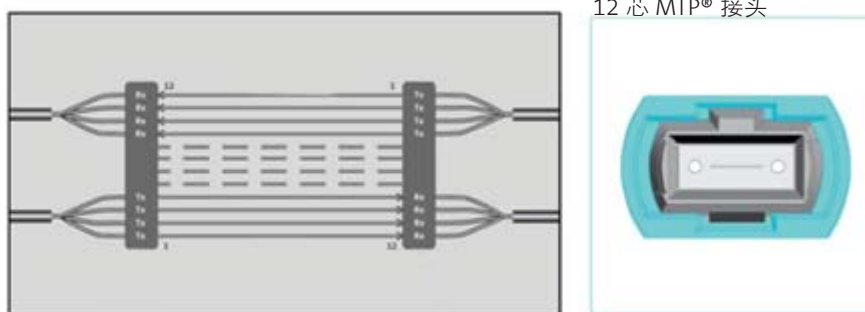
图 2: 并行多光纤(8 芯)光学传输
