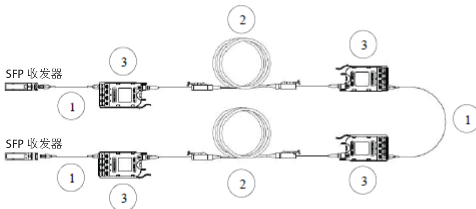
图 9: 使用交叉互联结构化布线的双光纤连接
