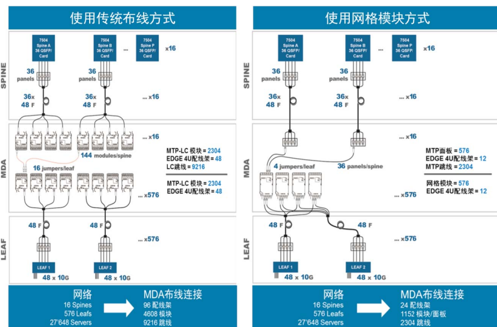
图 4: 脊叶两层网络结构 MDA 全交叉互联布线结构对比
