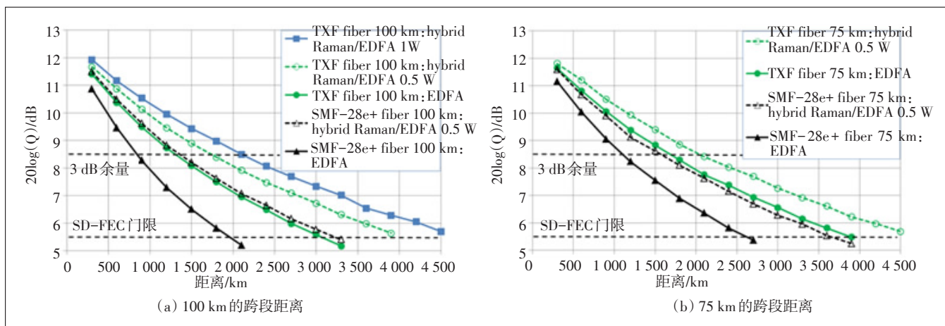
图2 16QAM的400G系统Q因子与传输距离的关系
