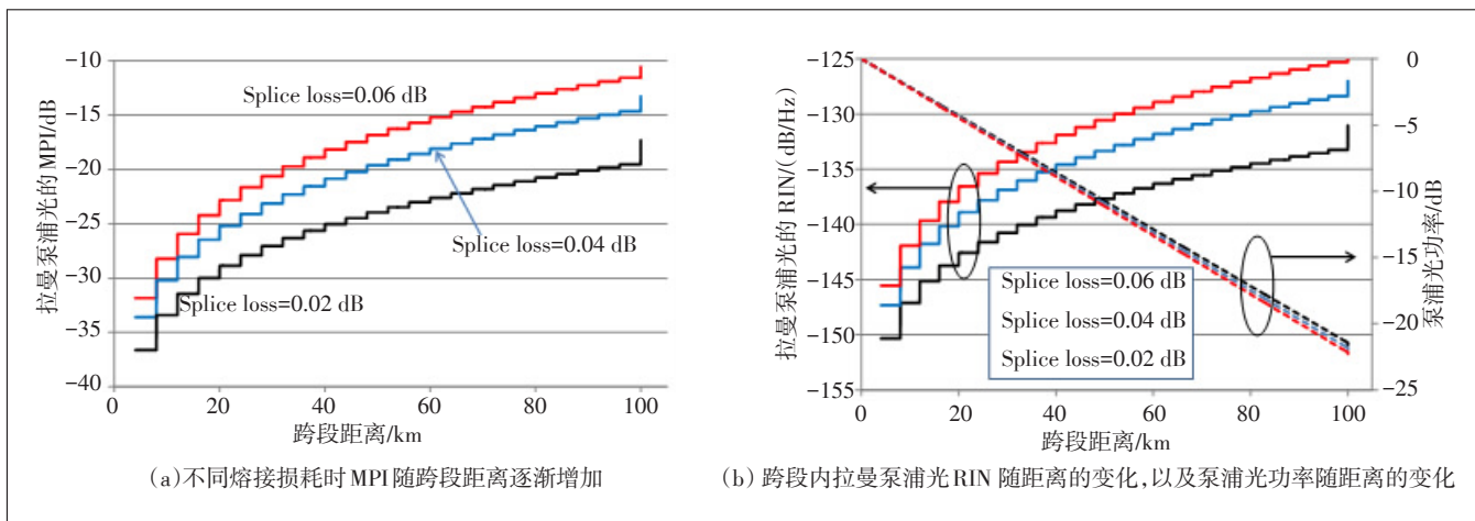
图3 MPI模型的结果
