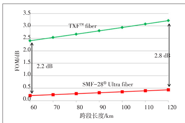
图1 G.654E、低损耗G.652D与常规G.652D光纤的FOM比较
