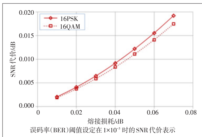
图 4 MPI 导致的泵浦光 RIN 对信号的损伤
