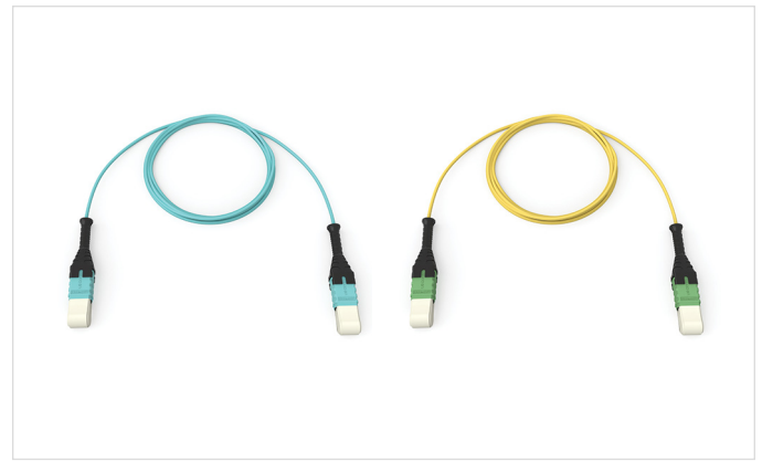
EDGE8 MTP Patchkabel | Fotos REN7928 und REN7927
