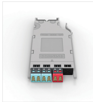
EDGE8 LC zu LC TAP Modul Foto REN3237
