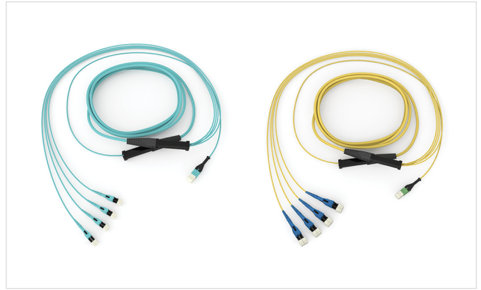
EDGE8 Hybrid MTP zu LC Uniboot Trunks | Fotos REN7958 und REN7957
