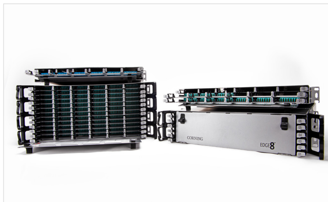
Vorbestückte EDGE8 Gehäuse | Foto CRR6147
