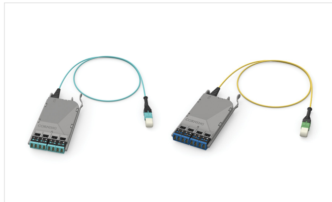
EDGE8 Port Breakout Module | Fotos REN7932 und REN7966
