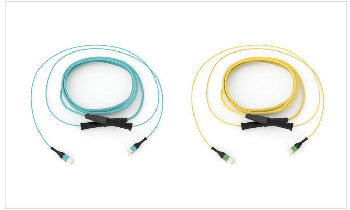
EDGE8 8-Faser MTP Extender Trunks | Fotos REN7954 und REN7953
