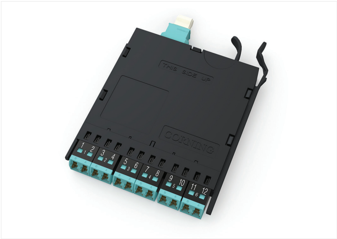
EDGE Module | Photo REN6521
