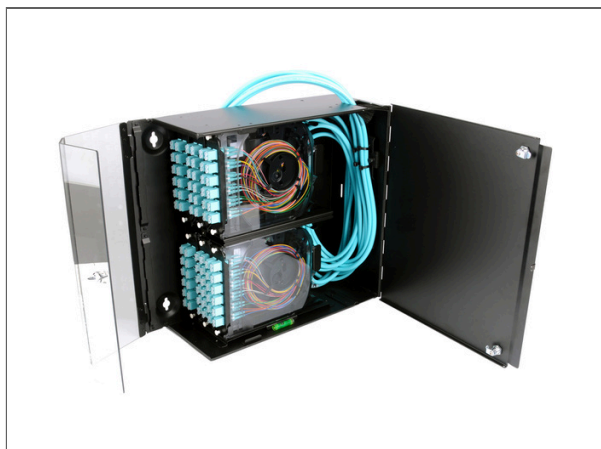
Carcasa de armario para montaje en la pared (WCH), contiene 6 paneles/casets de conectores CCH
