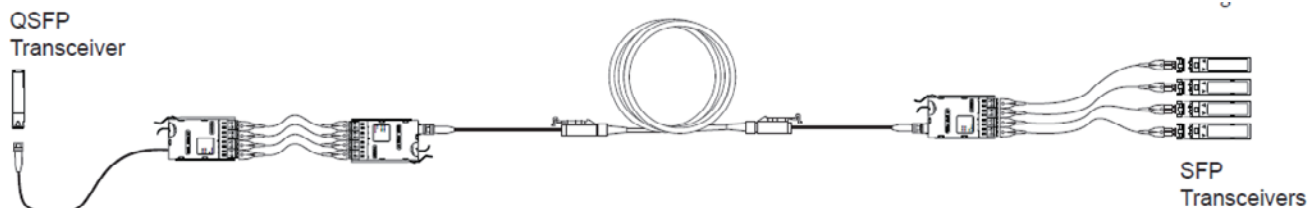
图 9c 一个交叉互连网络中，使用 8 芯端口分支预端接模块的端口分支
