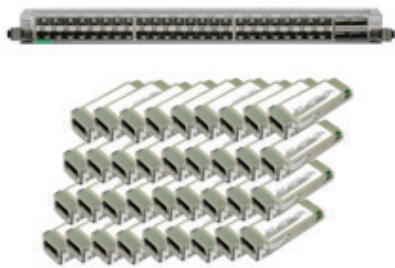
图 3. 48x10G SFP+ 线卡
