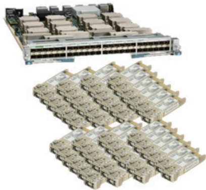
图 4. 36x40G QSFP 线卡
