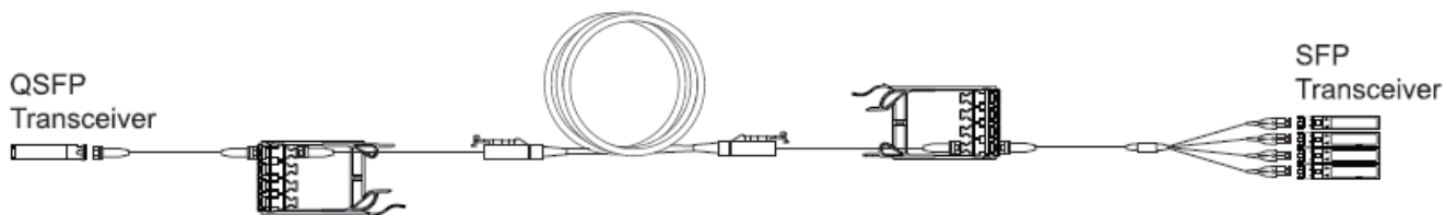
图 9a 使用 8 芯分支跳线的端口分支
