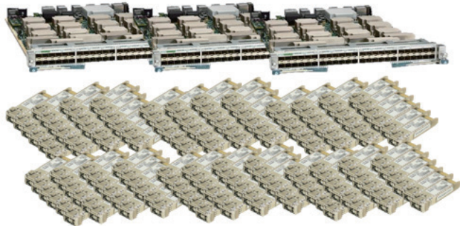
图 5. SFP+ 线卡和支持 144x10G 连接的收发器模块
