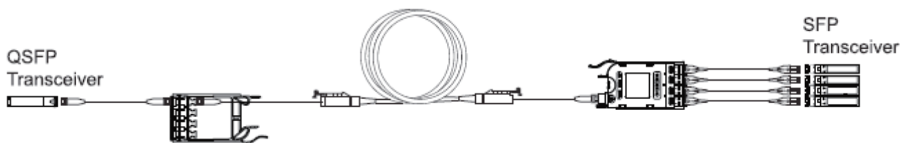
图 9b 使用 8 芯预端接模块的端口分支
