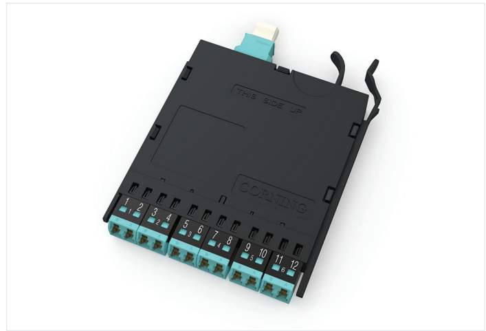
EDGE Module | Photo REN6521
